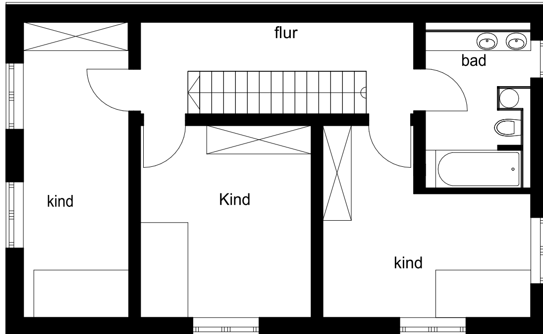
grundriss obergeschoss
